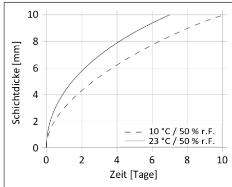
Diagramm 1: Durchhärtengeschwindigkeit von Sikaflex®-271
